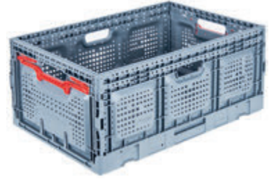
PG-6426 En/W Boy/L Yükseklik Dış / Ext 400 x 600 x 259 mm İç / Int 376 x 576 x 251 mm Katlanmış Yükseklik 47 mm Folded Height 47 mm
