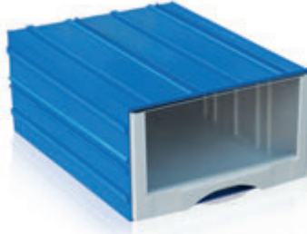
501-G En/W Boy/L Yük/H Dış / Ext 212 x 306 x 128 mm İç / Int 193 x 290 x 110 mm
