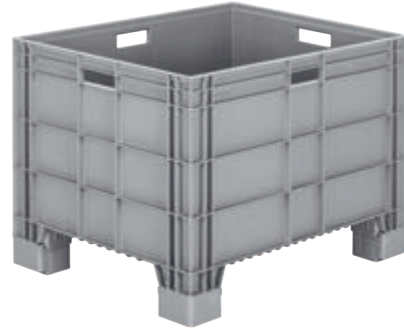
Kod / Code AX-8650-X En/W Boy/L Yük/H Dış / Ext 600 x 800 x 580 mm İç / Int 565 x 760 x 435 mm
