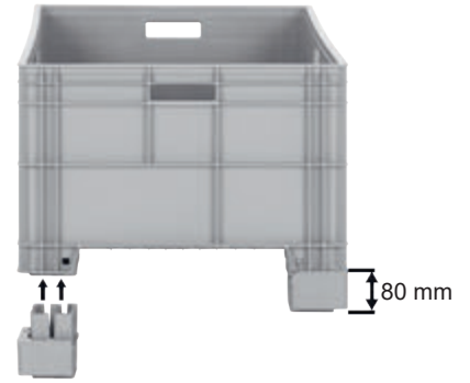
Kod / Code AX-86 AYK En/W Boy/L Yük/H Dış / Ext 60 x 50 x 80 mm AX-8650 ve AX-8639 uyumlu 80 mm yükseltme takozu, transpalet ve forkliftle kullanılmasını sağlar. 80 mm rising wedges are compatible with AX-8650 and AX-8639 and are used to make crates compatible with transpallet and forklift
