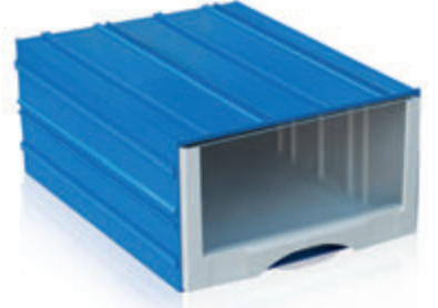
511 En/W Boy/L Yük/H Dış / Ext 260 x 340 x 150 mm İç / Int 246 x 325 x 135 mm
