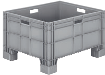
Kod / Code AX-8639-X En/W Boy/L Yük/H Dış / Ext 600 x 800 x 470 mm İç / Int 565 x 760 x 330 mm
