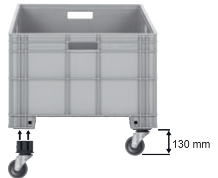
Kod / Code AX-86-T En/W Boy/L Yük/H Dış / Ext 60 x 50 x 130 mm AX-8650 ve AX-8639 uyumlu teker. Compatible wheels for AX-8650 and Ax-8639
