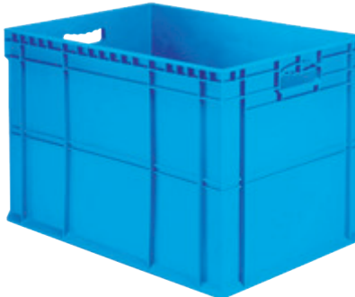
Kod / Code HP-4203 En/W Boy/L Yükseklik Dış / Ext 400 x 600 x 425 mm İç / Int 365 x 565 x 410 mm
