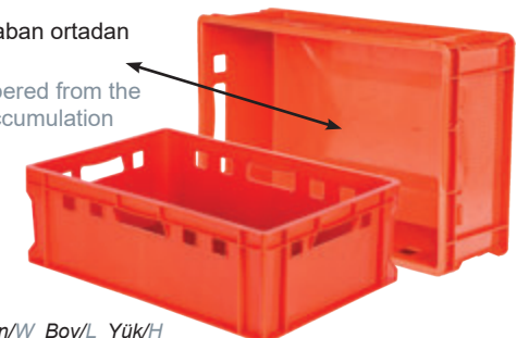
En/W Boy/L Yükseklik Dış / Ext 400 x 600 x 200 mm İç / Int 370 x 570 x 110 mm
