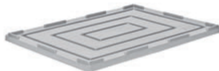
Kod / Code AX-8650-T En/W Boy/L Yük/H Dış / Ext 600 x 800 x 630 mm İç / Int 565 x 760 x 435 mm
