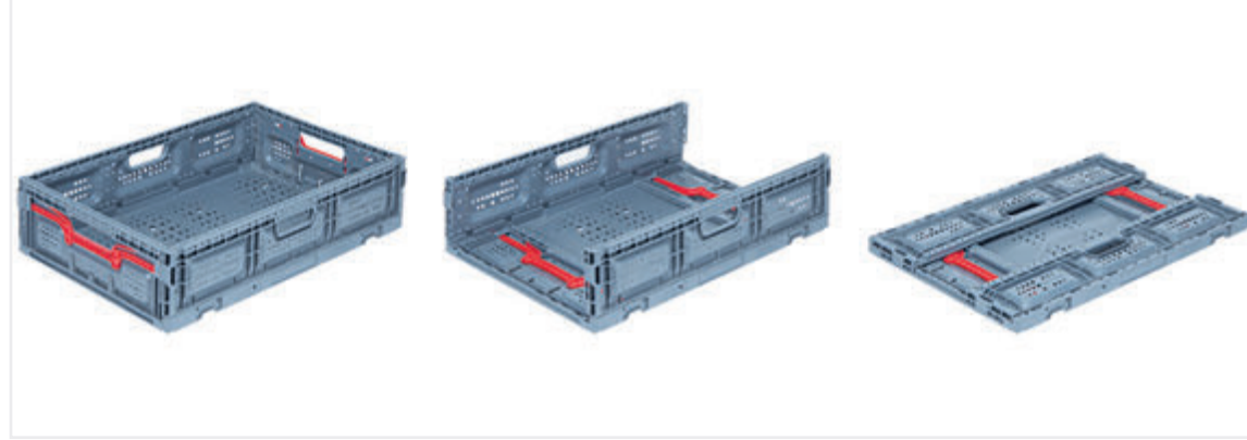
PG-6426 En/W Boy/L Yükseklik Dış / Ext 400 x 600 x 259 mm İç / Int 376 x 576 x 251 mm Katlanmış Yükseklik 47 mm Folded Height 47 mm
