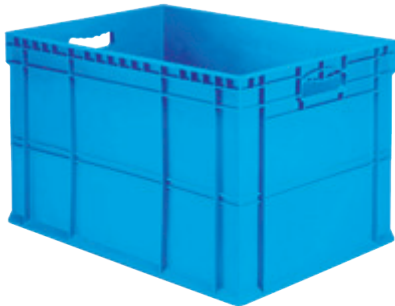
Kod / Code HP-3603 En/W Boy/L Yükseklik Dış / Ext 400 x 600 x 360 mm İç / Int 365 x 565 x 342 mm
