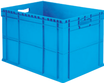
Kod / Code HP-4003 En/W Boy/L Yükseklik Dış / Ext 400 x 600 x 400 mm İç / Int 365 x 565 x 386 mm
