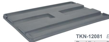
HP-82x120 En/W Boy/L Yüksek/H Dış / Ext 805 x 1270 x 60 mm K-550 uyumlu kapak Lid for K-550
